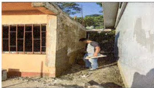
FOTO 11: Repello en muro aula 4
